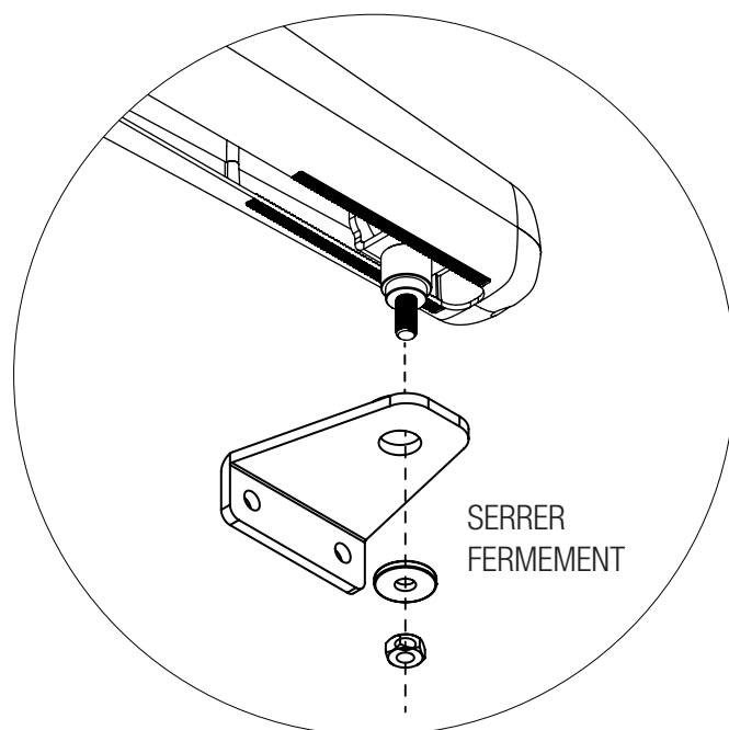
Fig. 8 ATTENTION! Lubrifier avec du gras le trou sur le support antérieure et l'écrou du moteur avant de le fixer.
